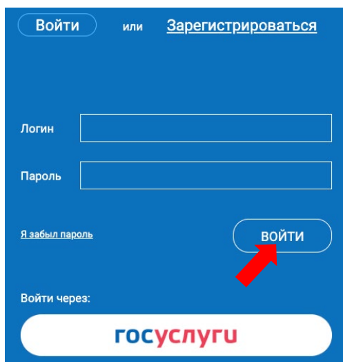
Рисунок 11 – Экран авторизации
