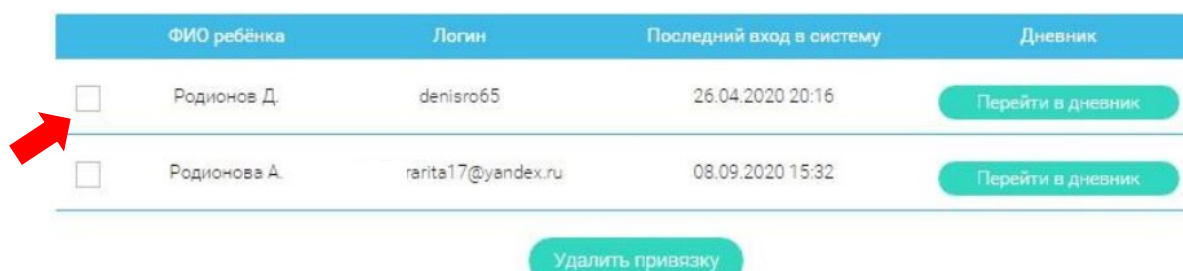
Рисунок 53 - Привязка учеников
