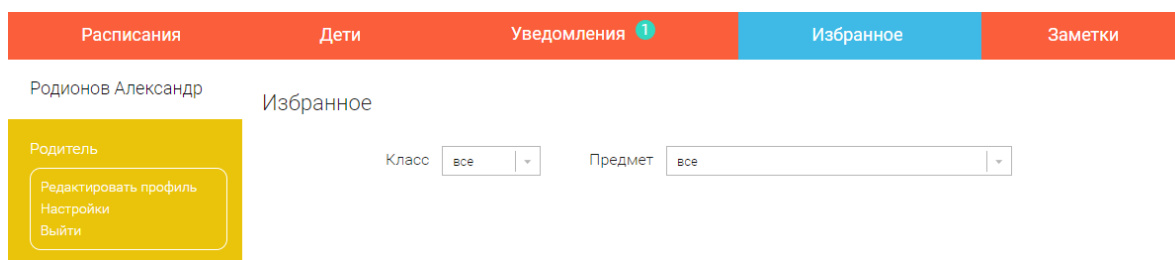
Рисунок 34 – Раздел «Избранное»
