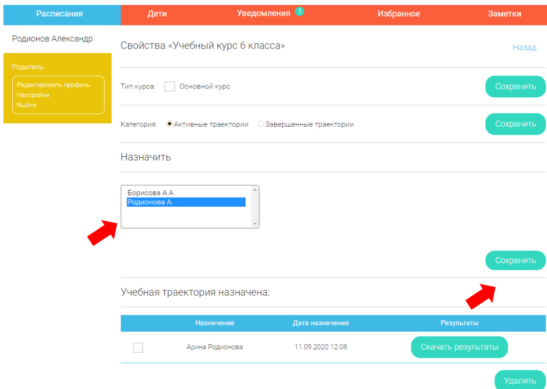
Рисунок 51 - Свойства траектории
