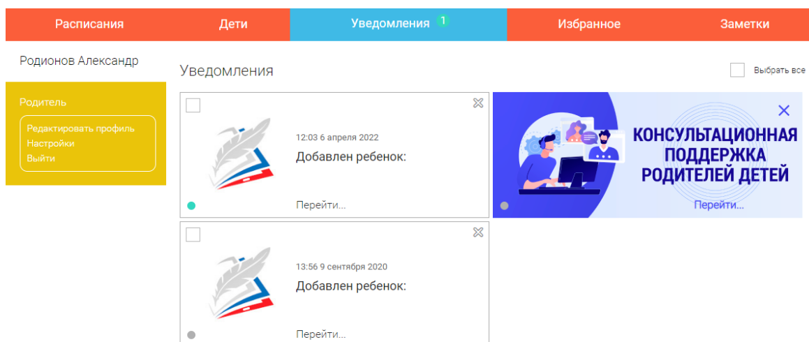
Рисунок 33 – Вкладка «Уведомления»
