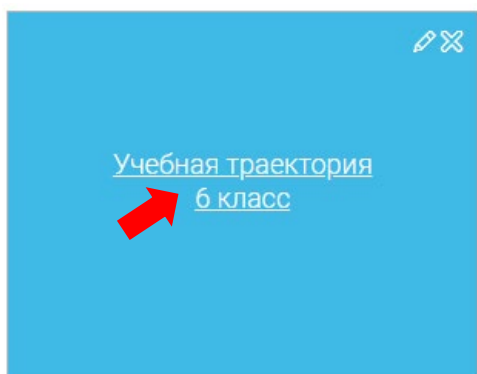
Рисунок 44 - Учебная траектория
